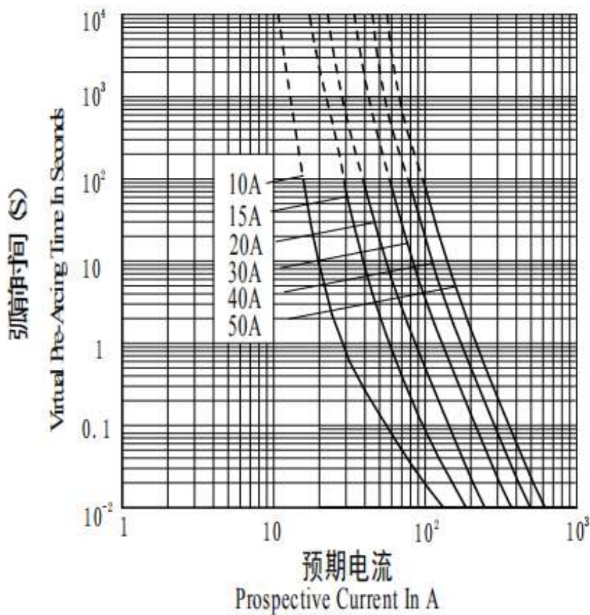
时间-电流特性曲线图
